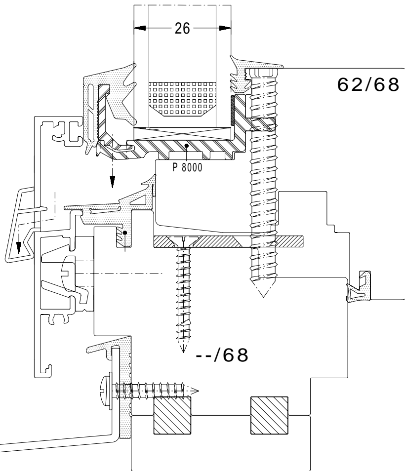
3-fach Verglasung ohne Glasfalzänderung
