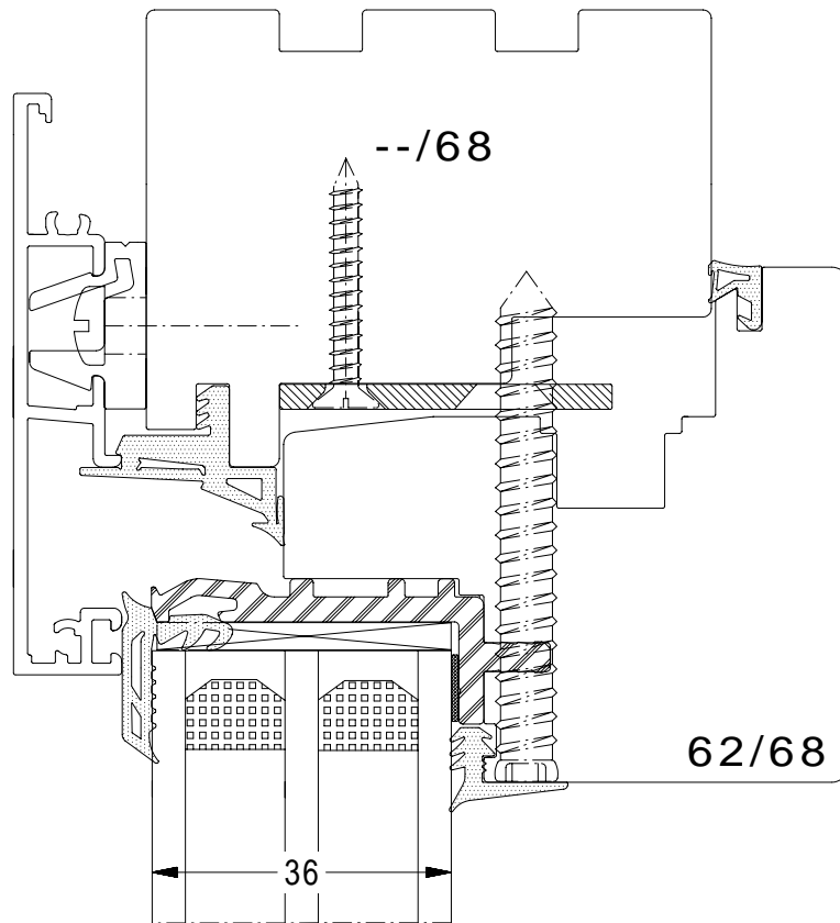
3-fach Verglasung ohne Glasfalzänderung
