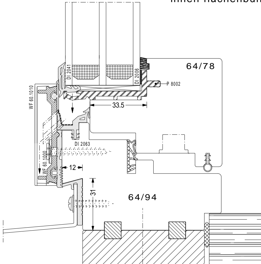
WF-VARIO LUX Integral-Ifb "innen flächenbündig"
